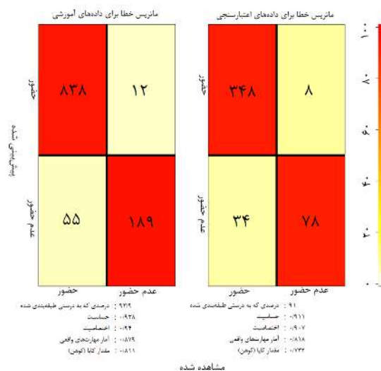
شکل ۵: ماتریس خطا برای داده‌های آموزشی و داده‌های اعتبارسنجی متقابل مطلوبیت زیستگاه J. excelsa روش رگرسیون تطبیقی چند متغیره اسپیلاین
